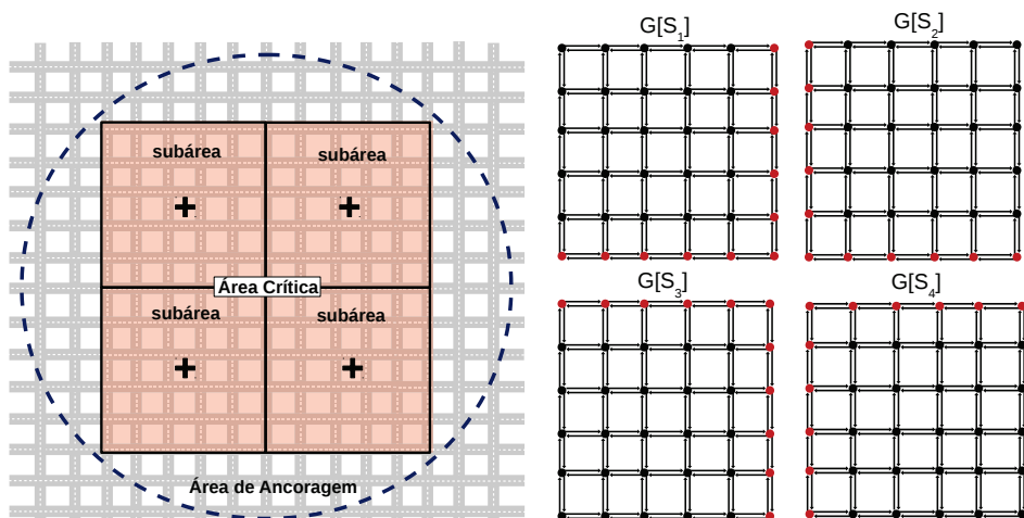
(a) Áreas de ancoragem, área crítica, k -subáreas e seus respectivos centros (b) Subgrafo induzido pelas arestas de cada subárea.
