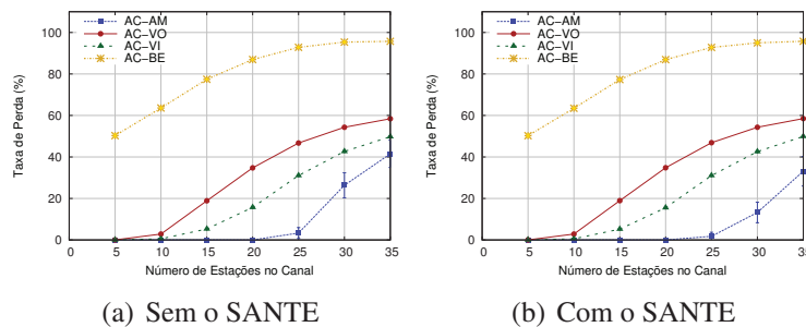
Figura 6. Taxa de Perda versus Densidade da Rede
