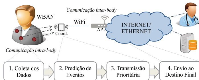
Figura 1. Arquitetura Geral do SANTE
