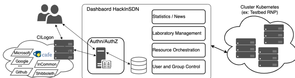
Figura 2. Arquitetura Dashboard HackInSDN.
