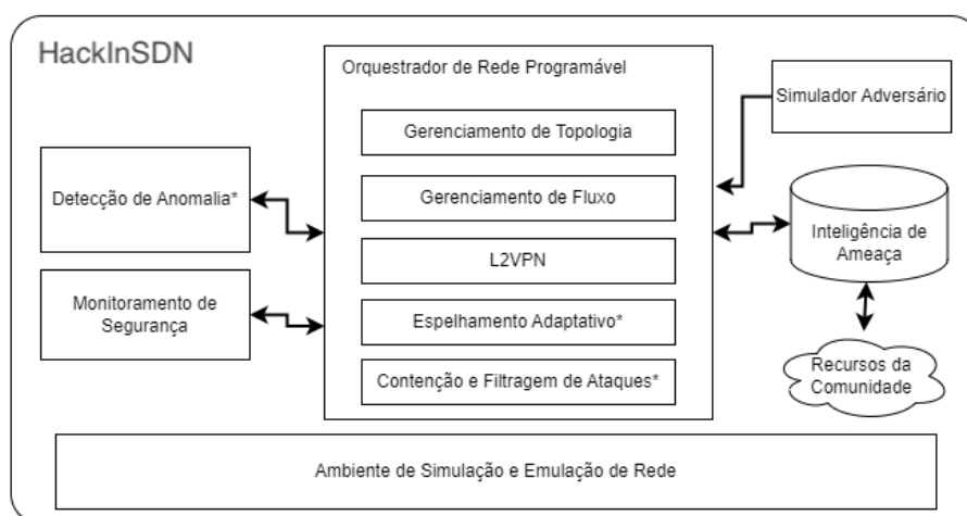
Figura 1. Módulos funcionais da arquitetura HackInSDN.
