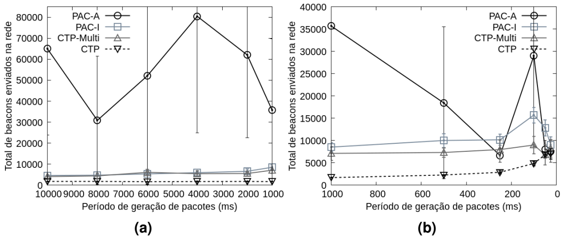
Figura 9. Gráficos que mostram a variação no número total de beacons com a mudança no período de geração de pacotes.
