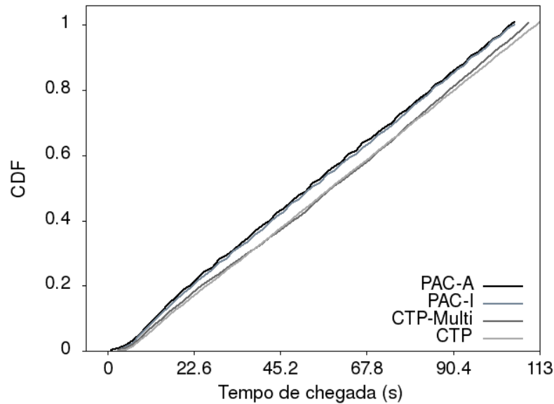
Figura 11. Gráfico da função de distribuição acumulada dos tempos de chegada das primeiras 2.000 mensagens.
