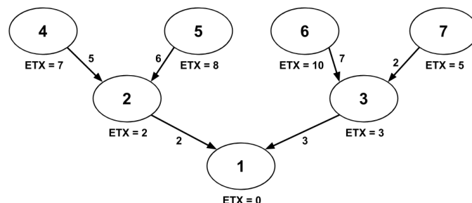
Figura 1. Exemplo de uma árvore formada pelo CTP, com os valores de ETX dos nós e dos enlaces.
