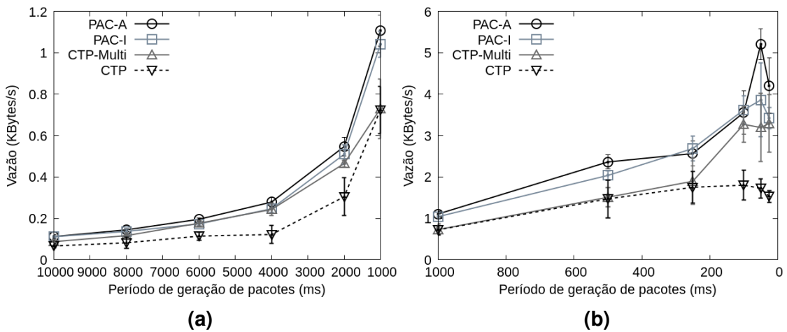
Figura 8. Gráficos que mostram a variação da vazão com a mudança no período de geração de pacotes.
