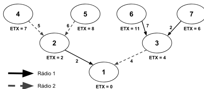
Figura 5. Exemplo da árvore formada pelo PAC-A, com os valores de ETX dos nós e dos enlaces para seus respectivos rádios.
