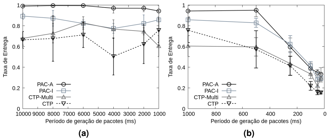
Figura 7. Gráficos que mostram a variação da taxa de entrega com a mudança no período de geração de pacotes.
