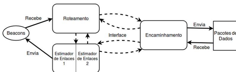
Figura 6. Esquema que ilustra as associações entre os principais componentes do PAC-A.
