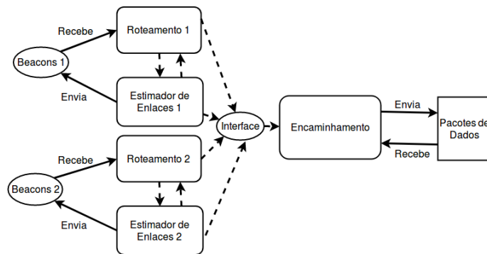
Figura 3. Esquema que ilustra as associações entre os principais componentes do PAC-I.
