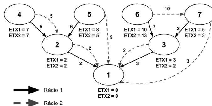
Figura 4. Exemplo das duas árvores formadas pelo PAC-I, com os valores de ETX dos nós e dos enlaces para cada rádio.
