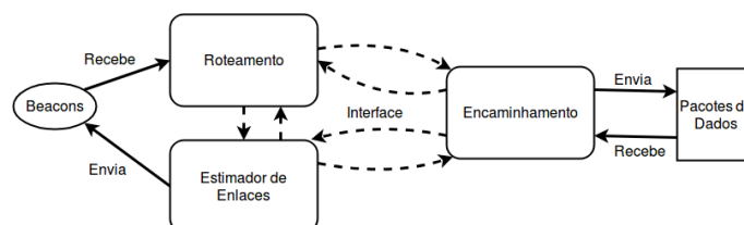
Figura 2. Esquema que ilustra as associações entre os três principais componentes do CTP.
