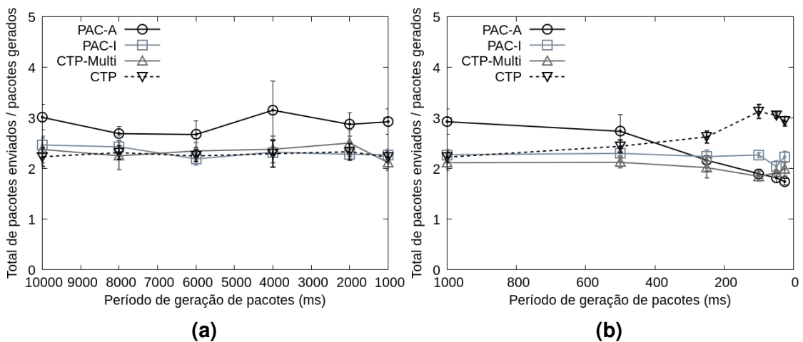
Figura 10. Gráficos que mostram a variação na razão do número total de pacotes de dados enviados na rede sobre o número de pacotes recebidos na raiz com a mudança no período de geração de pacotes.
