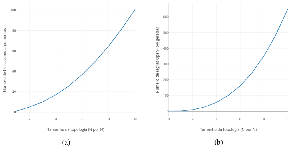
Figura 4. Gráficos com base no tamanho lateral da topologia.
