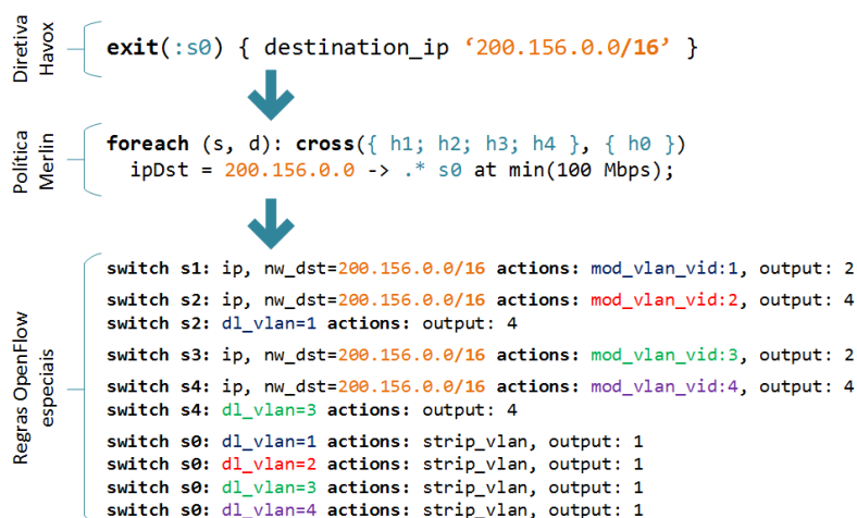
Figura 3. Transformação da diretiva em regras na topologia 2 por 2.
