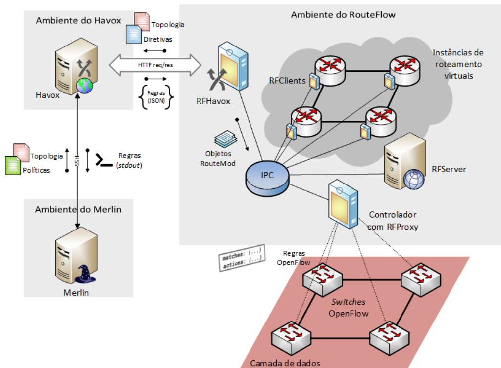
Figura 1. A arquitetura Havox.
