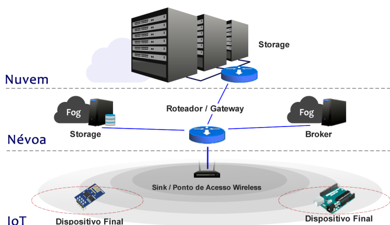
Figure 3. arquitetura de simulações do IoT FogSim.
