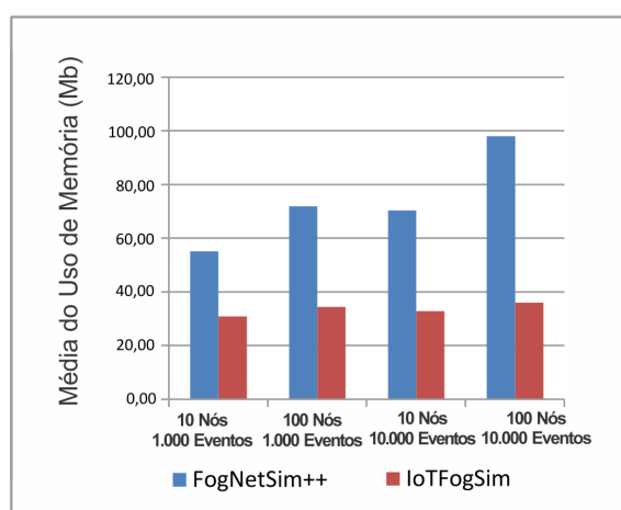
Figure 4. Comparação entre o uso de memória entre os simuladores.
