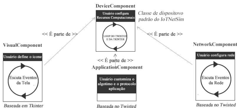
Figure 2. Arquitetura de um nó do simulador IoTFogSim.
