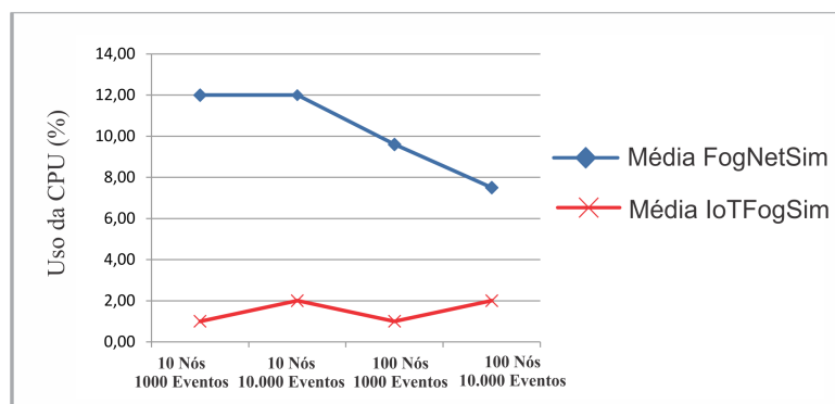
Figure 5. Comparação entre o uso de CPU entre os simuladores.
