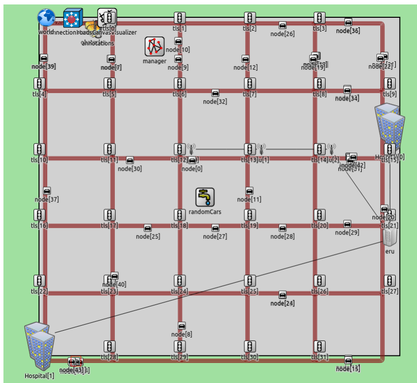
Figura 3. Grade simulada.
