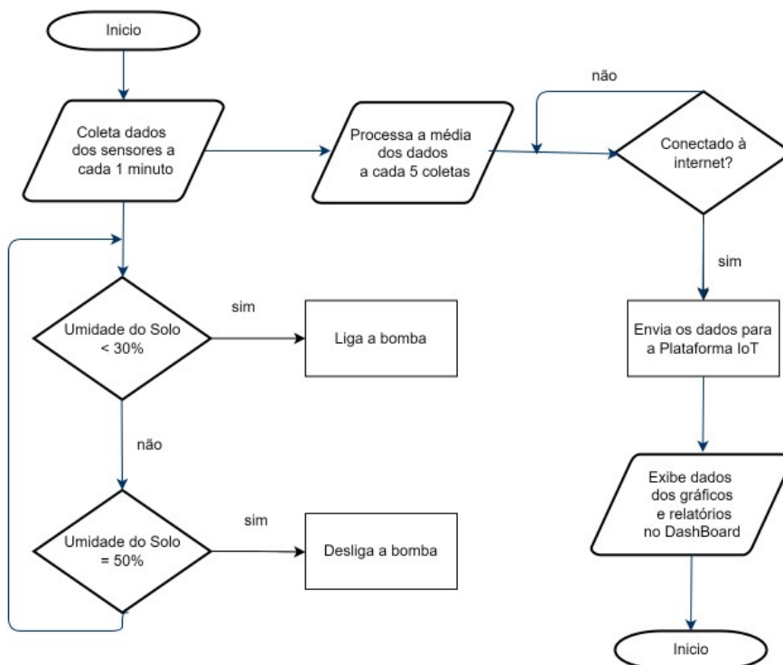
Figura 3. Fluxograma do funcionamento da solução
