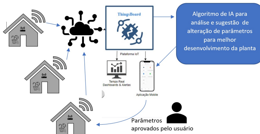
Figura 1. Modelo conceitual para a Internet social das Plantas
