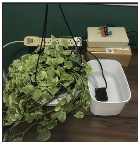
Figura 5. Protótipo SmartPlant.
