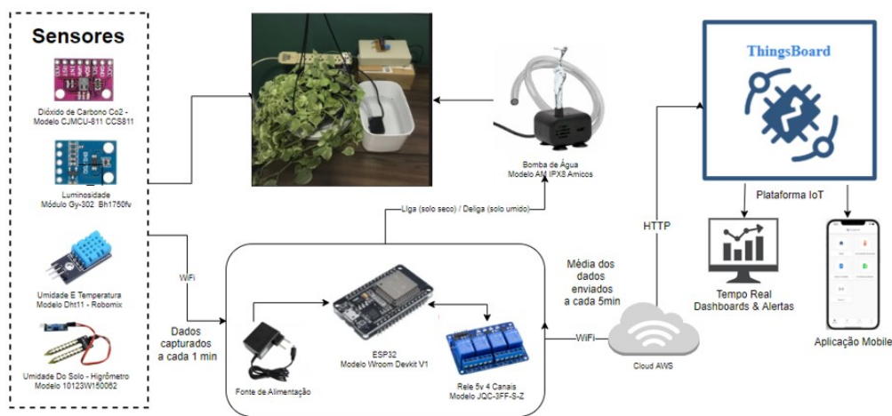
Figura 2. Diagrama contendo os principais elementos do protótipo SmartPlant.
