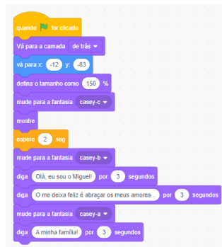
Figura 4: Código do personagem principal.
