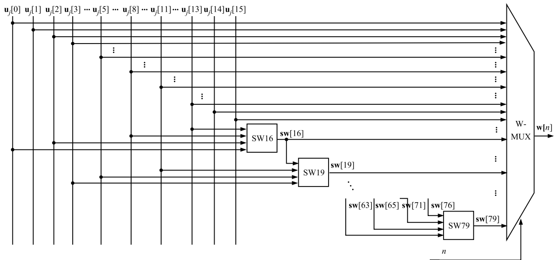
Figura 3. Arquitetura do módulo GW
