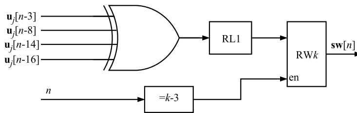
Figura 4. Operações do módulo SW_k
