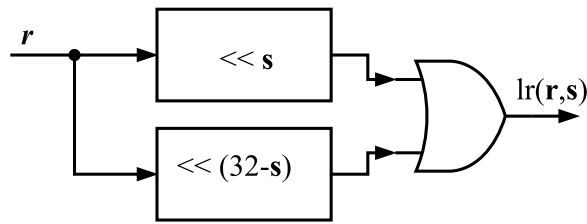
Figura 5. Arquitetura do módulo RL_s .
