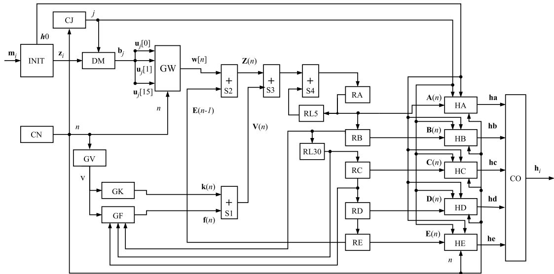
Figura 1. Arquitetura geral da implementação em hardware do SHA-1 proposto.
