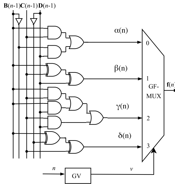
Figura 2. Arquitetura do módulo GF.
