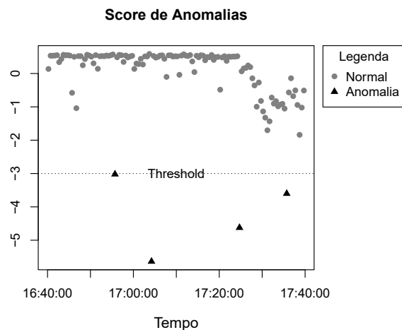
Figura 7. Score de anomalias gerado pelo IDS com parâmetros \delta = 1 e \sigma = 2^{-5}
