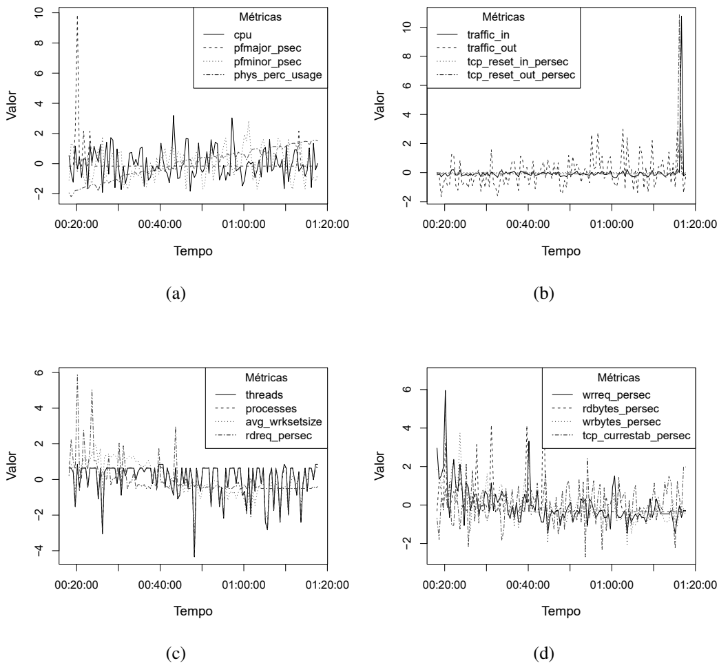
Figura 3. Perfil das métricas de desempenho durante um ataque de port scan agressivo
