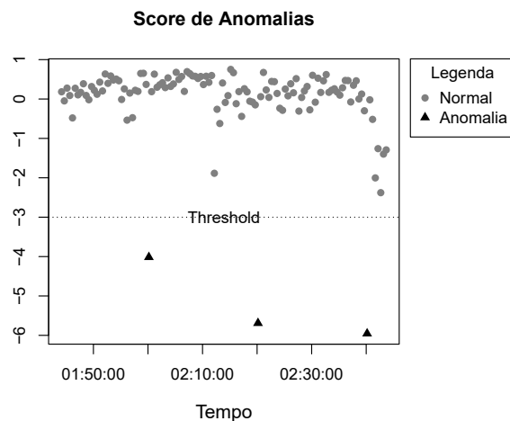
Figura 5. Score de anomalias gerado pelo IDS com parâmetros \delta = 1 e \sigma = 2^{-5}
