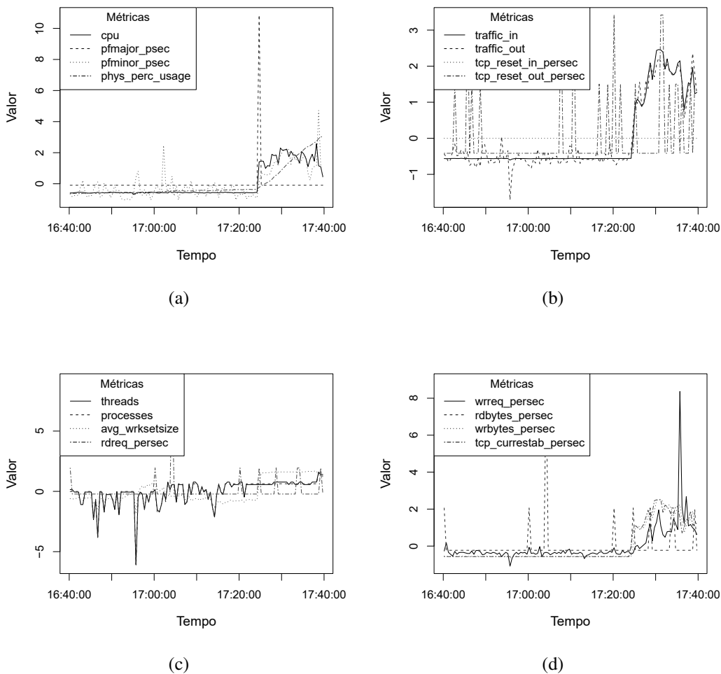
Figura 6. Perfil das métricas de desempenho durante um ataque de DDoS na camada de aplicação
