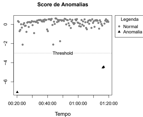
Figura 4. Score de anomalias gerado pelo IDS com parâmetros \delta = 1 e \sigma = 2^{-5}
