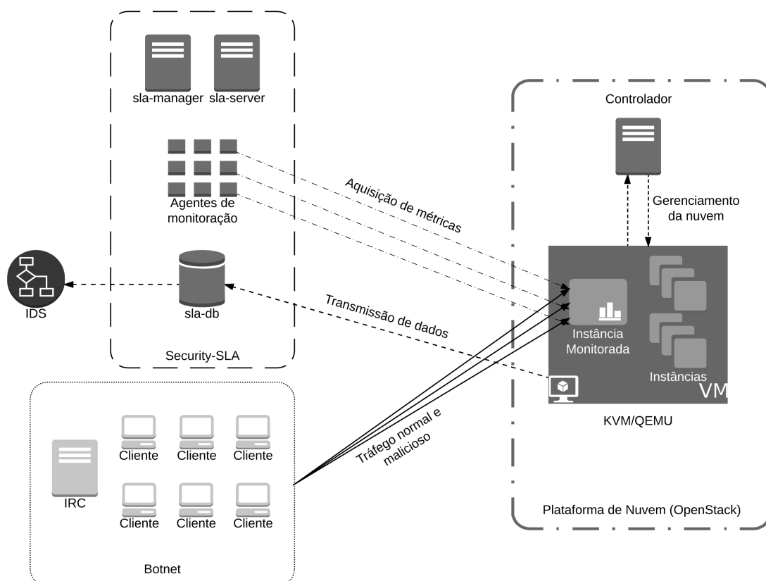
Figura 1. Arquitetura lógica do ambiente
