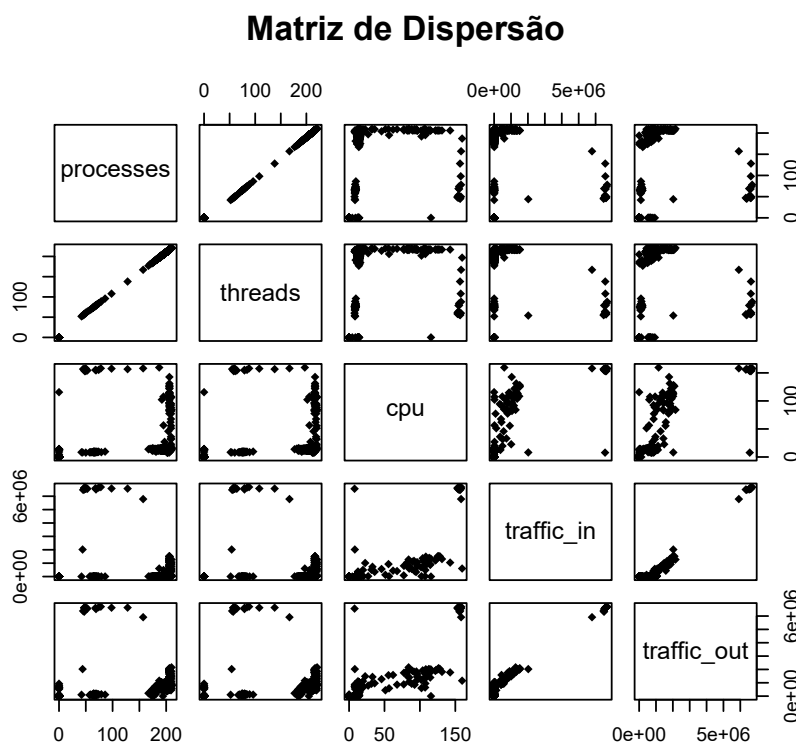
Figura 2. Matriz de dispersão das métricas processes , threads , cpu , traffic_in e traffic_out
