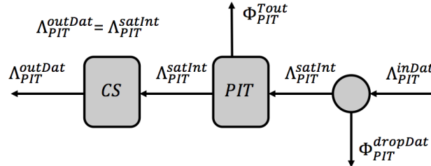
Figura 3. Processamento de Pacotes de Dados no CS e na PIT.
