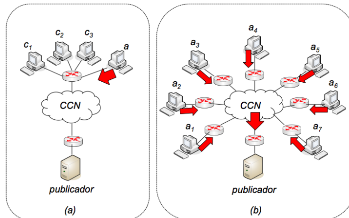
Figura 1. (a) Ataque de inundação ao roteador de borda dos consumidores e (b) Ataque de inundação ao roteador de borda do publicador.
