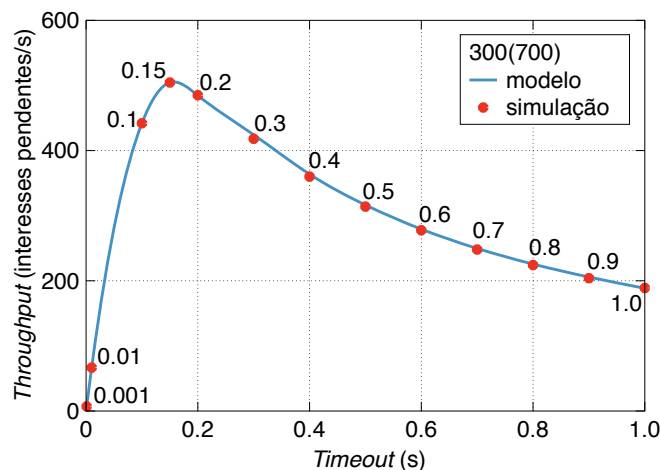
Figura 7. Comparação do modelo de otimização e simulação da taxa de interesses pendentes atendidos em função do valor do tempo máximo de permanência na PIT.
