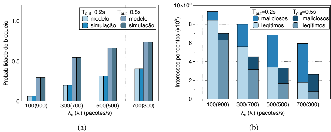
Figura 5. (a) Probabilidade de bloqueio x intensidade do tráfego malicioso e (b) Total de interesses pendentes legítimos e maliciosos armazenados na PIT.
