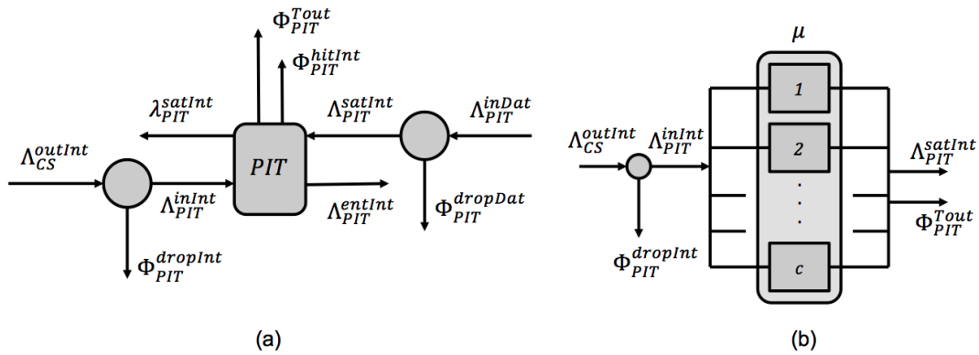
Figura 4. (a) Abstração da PIT e (b) Modelagem pelo sistema M/G/c/c.
