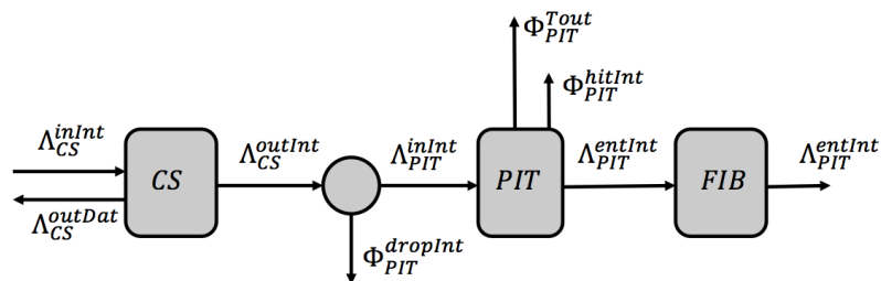
Figura 2. Processamento de Pacotes de Interesse no CS e na PIT.
