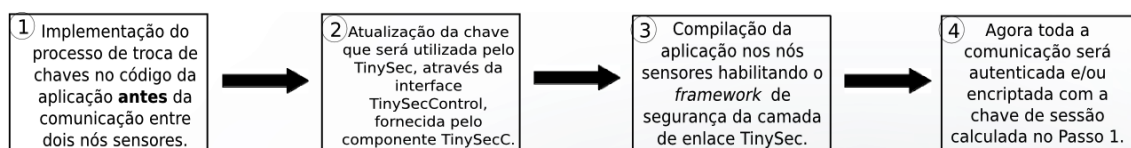
Figura 2. Descrição dos passos para utilização da nova abordagem de distribuição de chaves e o framework da camada de enlace TinySec
