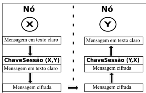
Figura 1. Envio da mensagem do nó X para o nó Y
