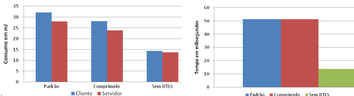
Figura 5. (a) Consumo de energia para um pacote de dados (b) Tempo total (RTT) no cliente
