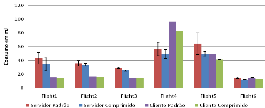
Figura 3 - Consumo de Energia por flight
