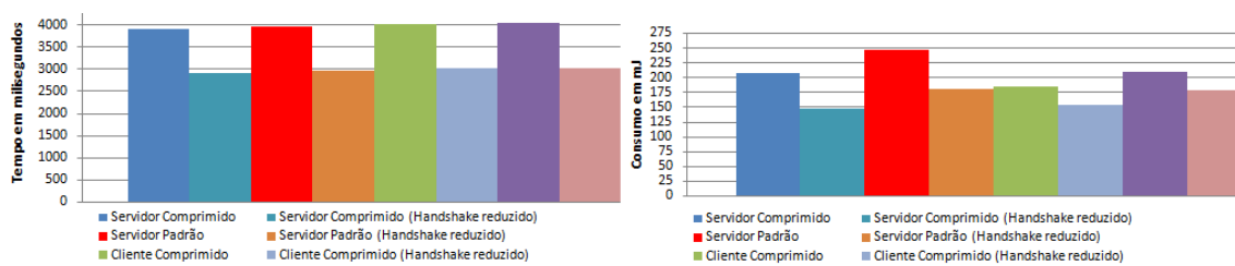
Figura 4. (a) Tempo total do handshake (b) Consumo total de energia do handshake
