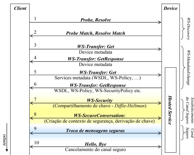
Figura 3. Estabelecimento de canais seguros
