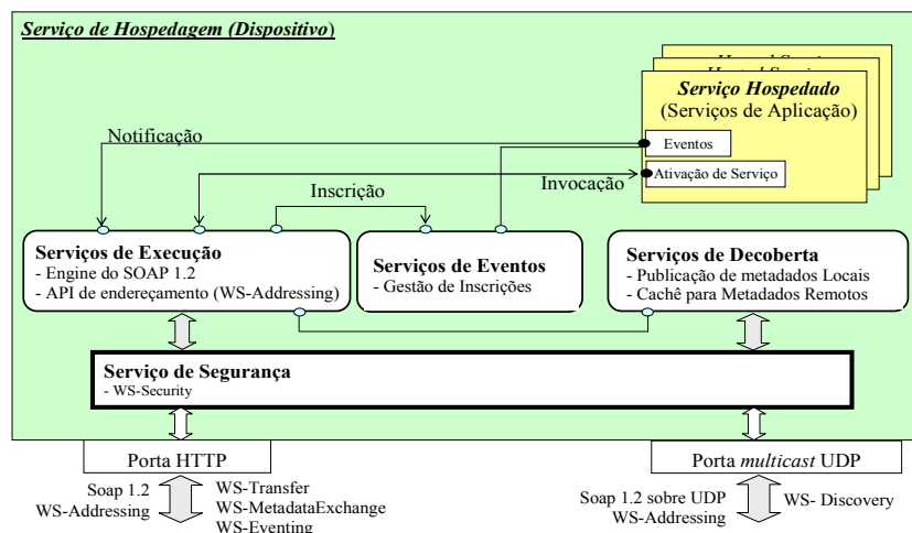
Figura 1. Modelo computacional do DPWS
