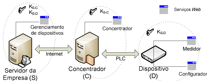
Figura 4 - Componentes e Serviços Web da aplicação alvo
