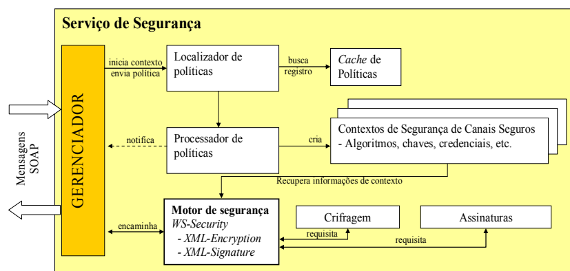
Figura 2. Funcionalidades do Serviço de Segurança
