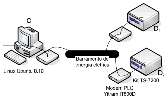
Figura 5. Configuração da rede para os ensaios.
