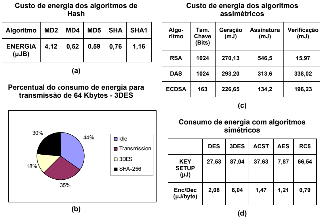
Figura 5: Gasto de energia com cifragem.
