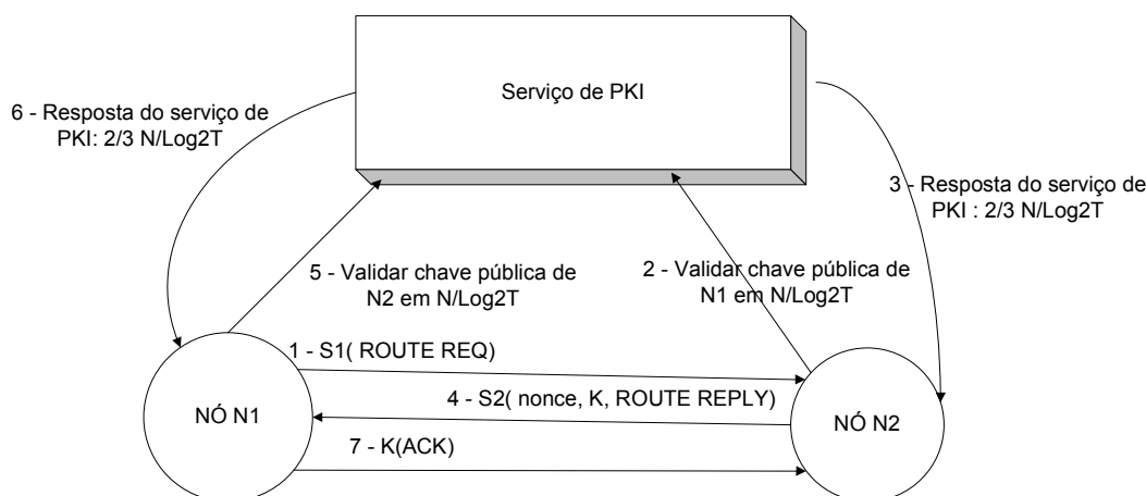
Figura 3: Protocolo de autenticação dos nós
