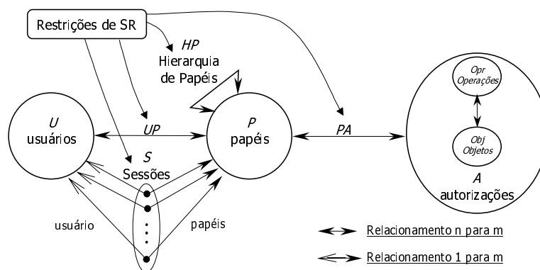
Figura 1 – Padrão NIST de referência para CABP (2)
