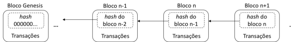
Figura 1: Visão esquemática da estrutura de dados em uma cadeia de blocos. O bloco genesis representa o primeiro bloco da cadeia. Cada bloco tem o resumo criptográfico do bloco anterior, gerando um encadeamento de resumos criptográficos. A alteração de um bloco gera a inconsistência de todos os blocos seguintes da cadeia.
