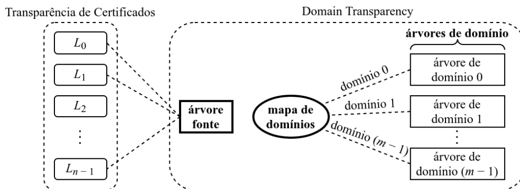
Figura 1. Visão geral de Transparência de Domínios. O mapa de domínios associa cada domínio a uma árvore de domínios e a árvore fonte lista os logs fonte. Cada árvore de domínio armazena, dentre todos os certificados presentes nos logs fonte, aqueles que estão associados ao seu domínio.
