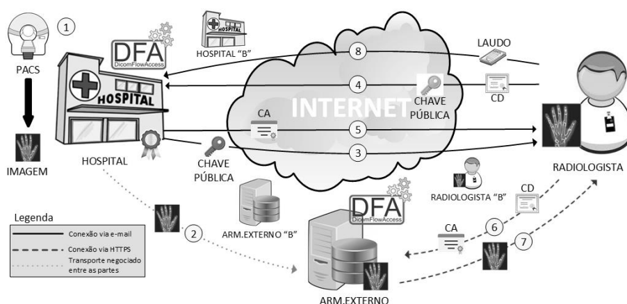
Figura 2: DICOMFlowAccess atuando como mecanismo de controle de acesso
