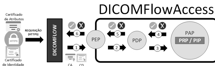
Figura 3: Funcionamento interno do DFA.
