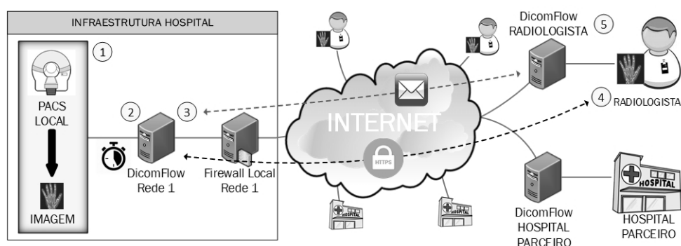
Figura 1: Rede de colaboração proposta pelo DicomFlow.
