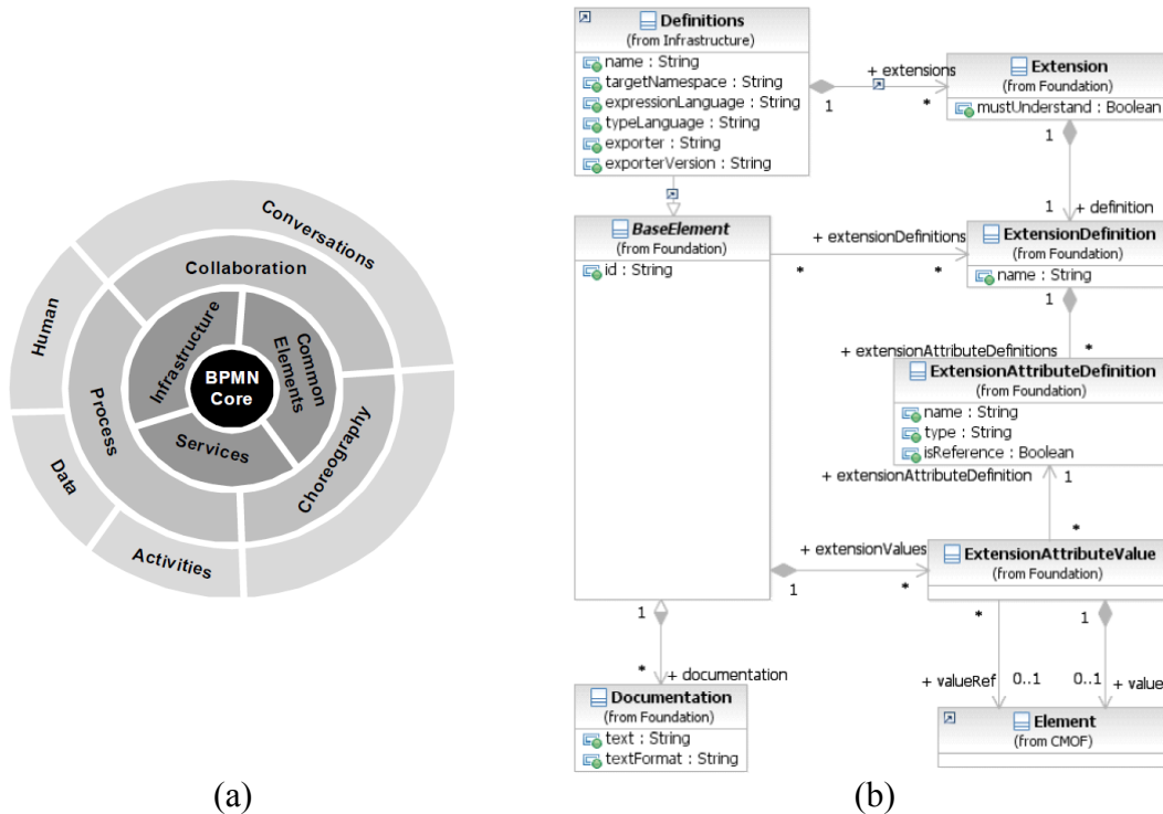
Figura 4: (a) Modelo de camadas do BPMN 2.0 (b) Conjunto de classes que definem o mecanismo de extensibilidade do BPMN 2.0
