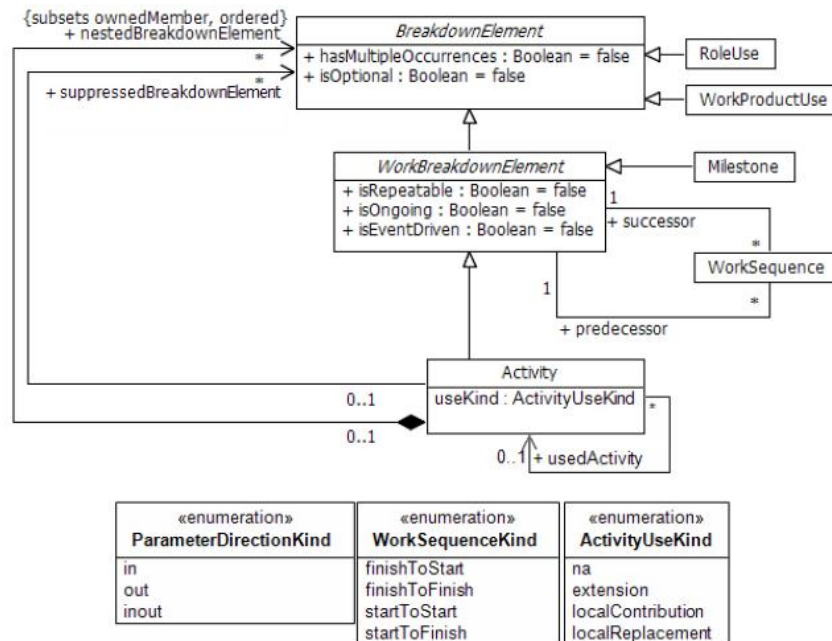
Figura 2: Modelo do pacote Process Structure
