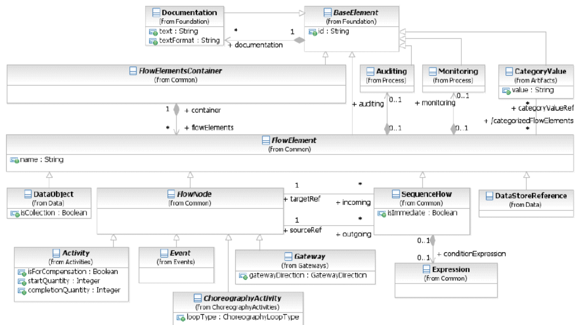
Figura 5: Diagrama de classes exibindo o relacionamento entre a classe BaseElement e as demais classes que compõem um Processo ou Coreografia
