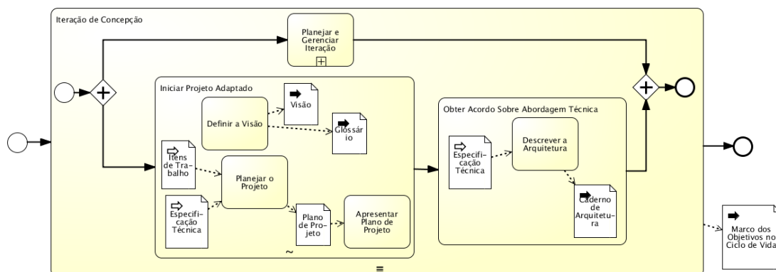
Figura 8: Processo final depois de realizado o tailoring
