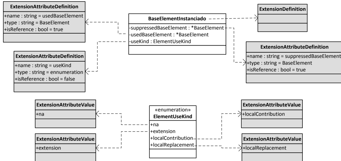
Figura 6: Representação da extensão proposta
