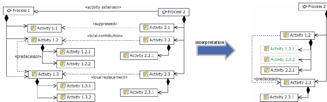
Figura 3: Ilustração do processo de reutilização previsto no SPEM 2.0
