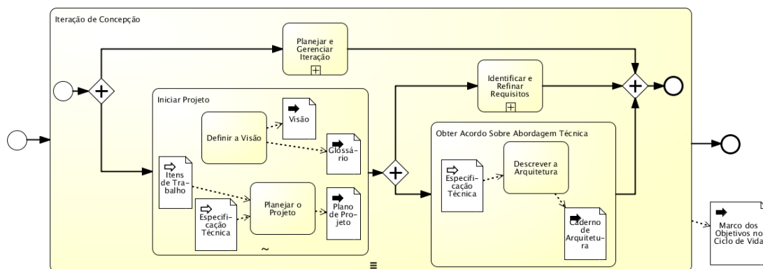
Figura 7: A fase de Concepção do Delivery Process do OpenUp
