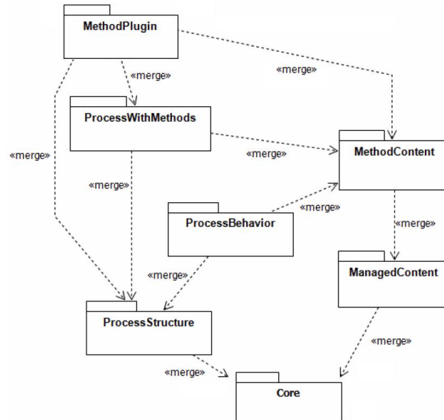
Figura 1: Divisão de pacotes do meta-modelo do SPEM
