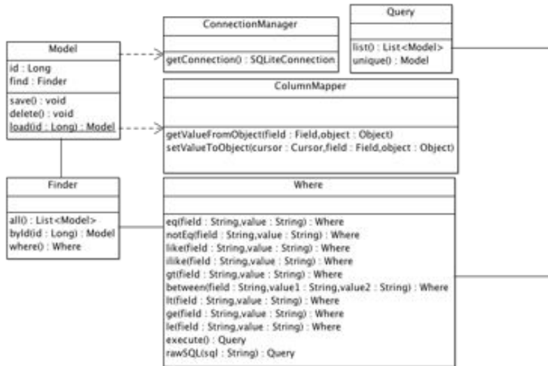
Figura 2. Diagrama de Classes
