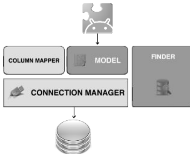
Figura 1. Arquitetura Interna do Aliendroid.
