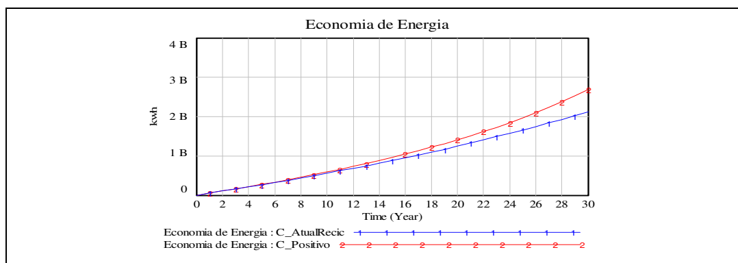
Figura 4. Economia de energia elétrica acumulada ao longo de 30 anos.
