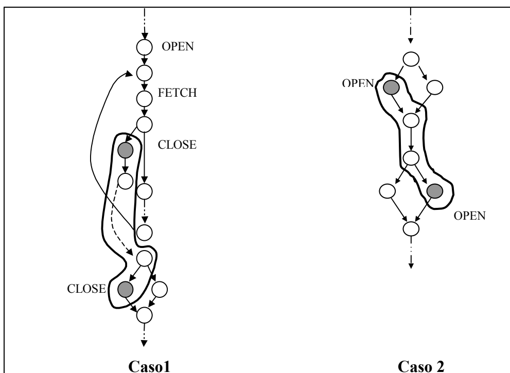
Figura 2. Exemplo de cenários de defeito para o uso de cursores
