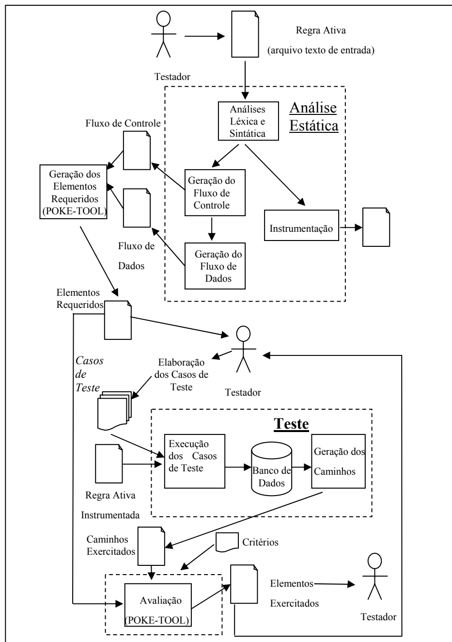
Figura 1. Arquitetura da ferramenta ART-TOOL.
