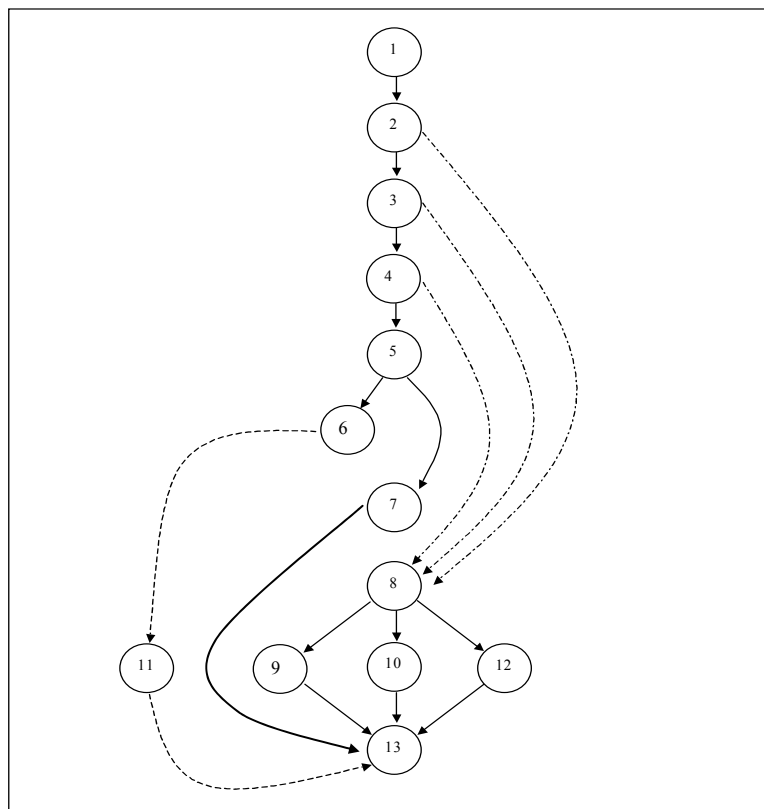
Figura 1. Representação do fluxo de controle da regra ativa R1
