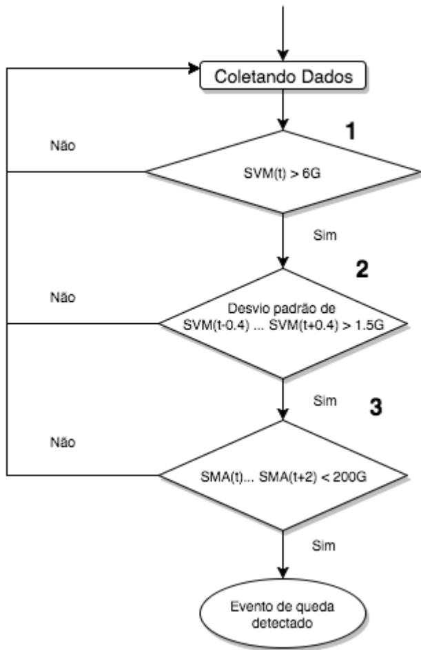
Figure 2: Fluxograma do algoritmo proposto. Figura Elaborada pelo autor (2016).
