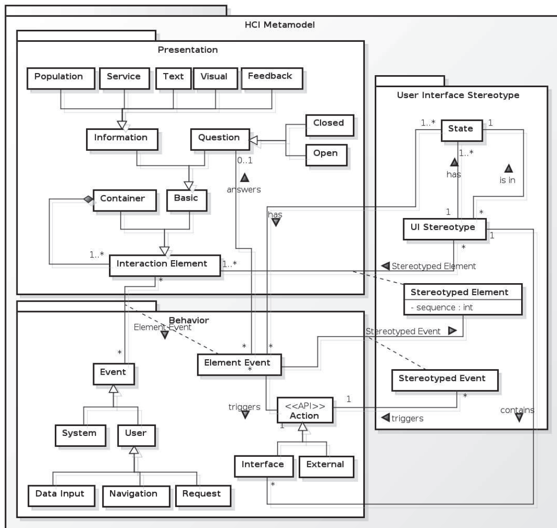
Figura 1. HCI Metamodel
