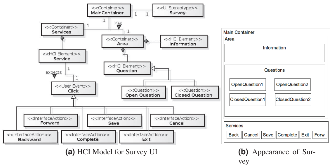
Figura 4. Survey UI Stereotype
