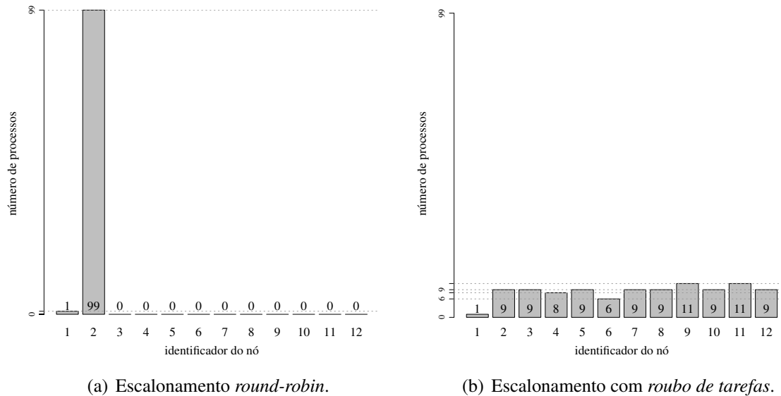
Figura 2. Balanceamento de carga de tarefas por nó usando dois algoritmos de escalonamento: round-robin , (a), e roubo de tarefas , (b).
