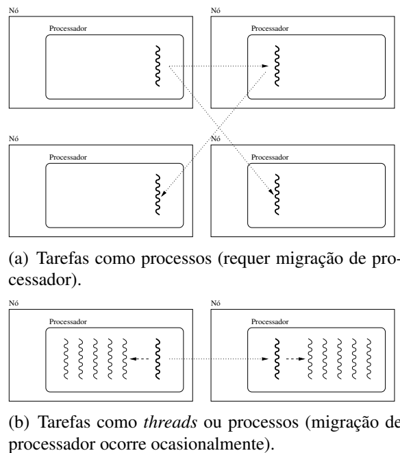
Figura 4. Aproveitamento de processadores disponíveis em \omega ciclos de clock sem o uso de controle de granularidade (a) e com o controle (b).
