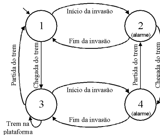
Figura 2: Estados e transições do sistema.
