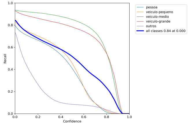
Figure 3. Gráfico referente a métrica Recall com a confiança
