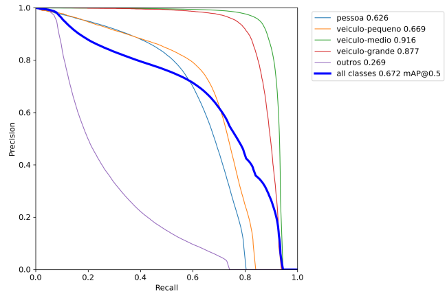
Figure 4. Gráfico referente a métrica Precision com a Recall formando a mAP
