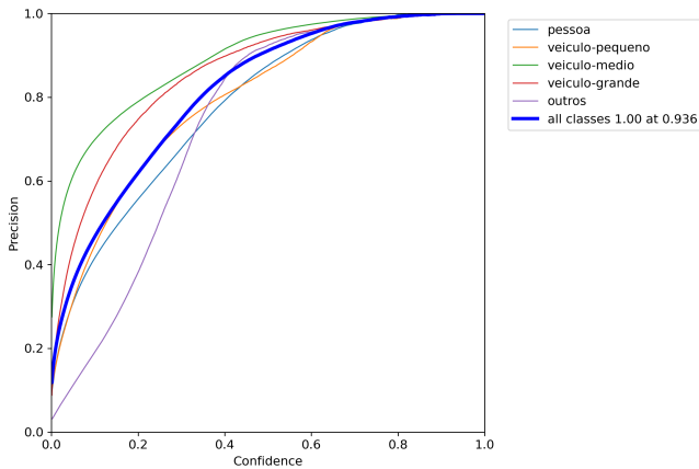
Figure 2. Gráfico referente a métrica Precision com a confiança
