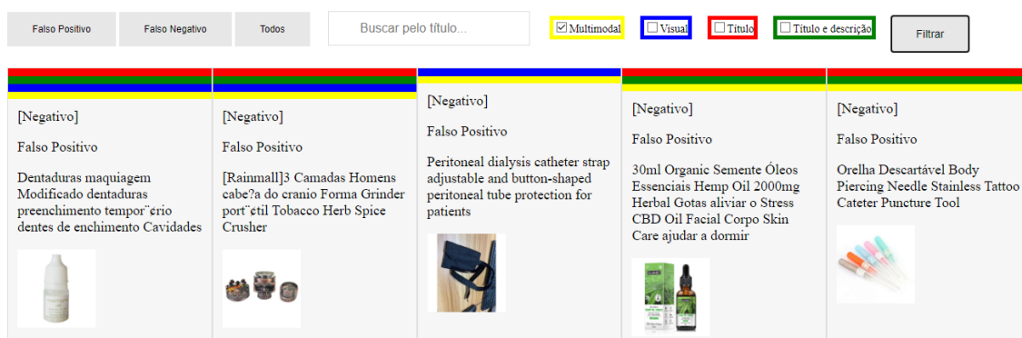
Figura 5. Interface desenvolvida para análise qualitativa dos erros de classificação dos modelos treinados ilustrando alguns falsos positivos.
