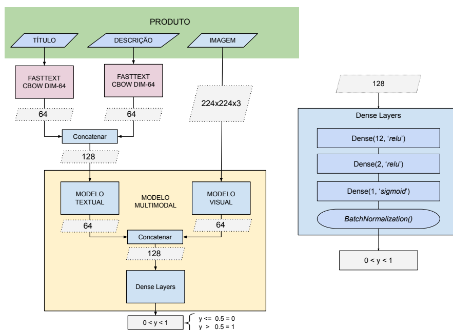
Figura 4. Descrição do modelo multimodal textual-visual produzido para este experimento.
