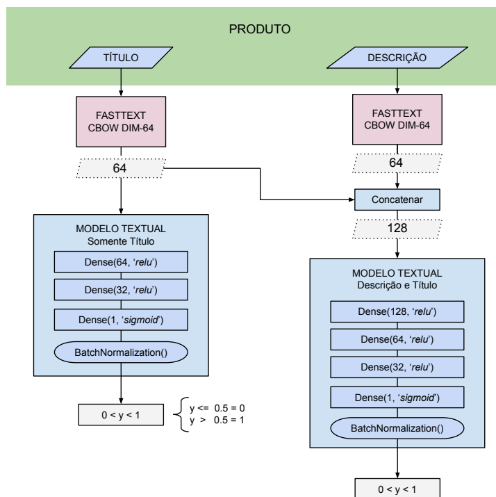
Figura 2. Descrição dos modelos unimodais textuais, onde a saída ( y ) representa a probabilidade do produto ser Adulto.
