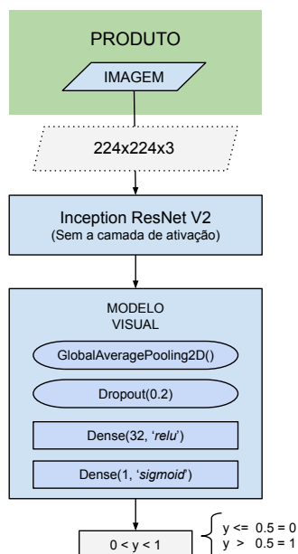
Figura 3. Descrição da combinação do modelo pré-treinado Inception ResNet V2 concatenado ao nosso modelo visual com função de ativação sigmoid .
