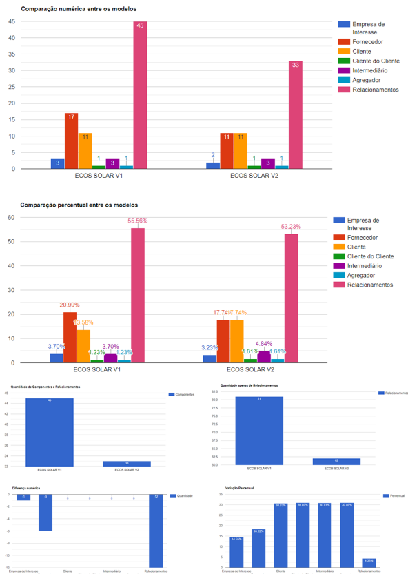
Figure 4: Gráficos com os resultados das comparações entre a versão 1 e 2 do ECOS SOLAR [4].
