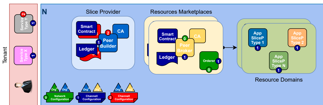
Figura 2. Modelo de arquitetura proposta para solução autônoma de monitoramento de SLA baseada no Hyperledger Fabric
