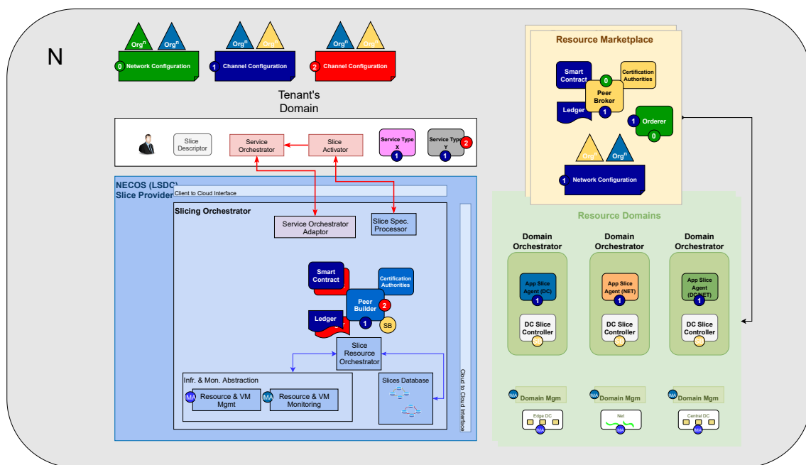
Figura 4. Modelo de arquitetura aplicada no cenário NECOS
