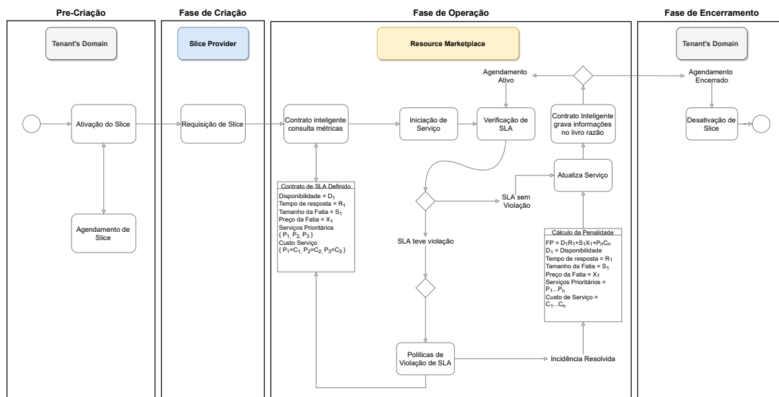
Figura 5. Fluxo de Monitoramento do Ciclo de Vida da Fatia
