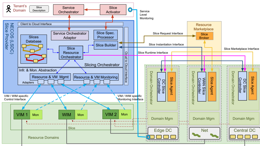
Figura 1. Arquitetura da plataforma [NECOS 2019]
