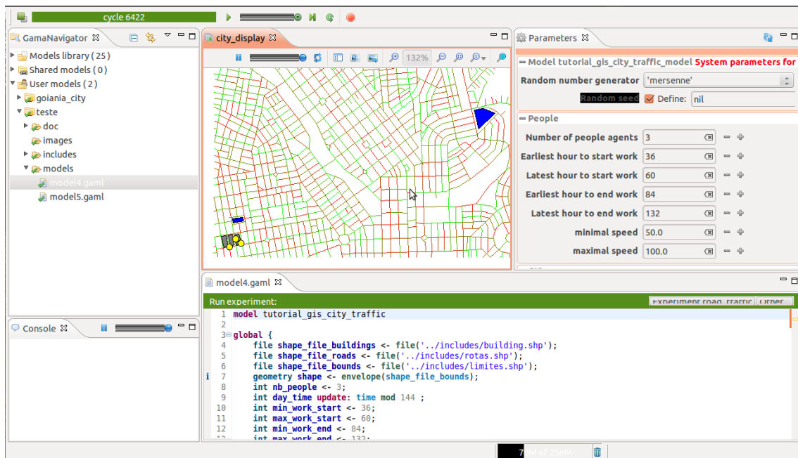
Figura 2. Simulação Multiagente no Projeto ADGEPA (3 agentes e uma grande área)
