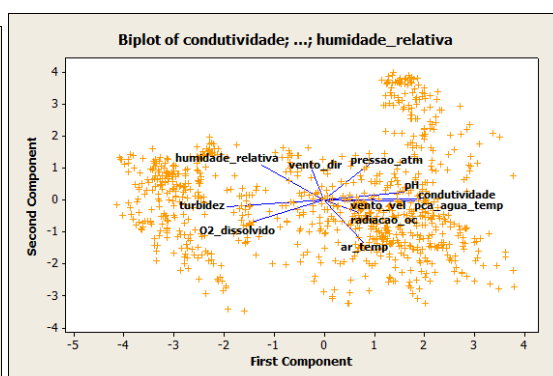
Figura 13. Gráfico integrado entre a carga dos fatores e o conjunto de dados
