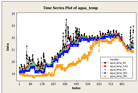
Figura 5. Série temporal dos dados de temperatura da água
