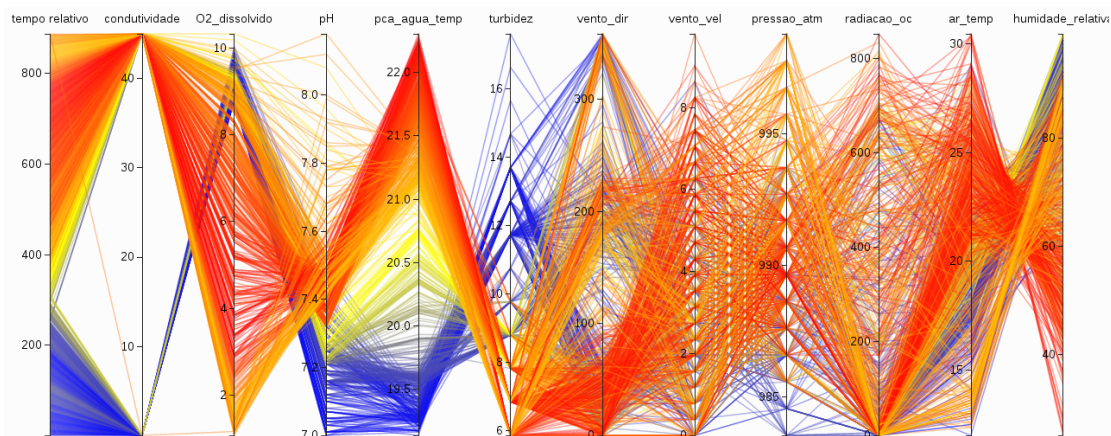
Figura 10. Representação em Coordenadas Paralelas dos dados selecionados
