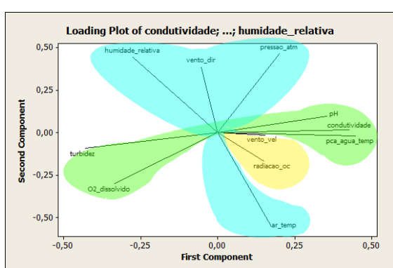
Figura 12. Relação de contribuição de cada variável nos PCs
