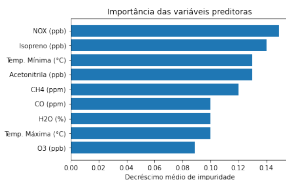
Figura 2. Importância de cada variável do modelo de Florestas Aleatórias para a espécie Coragyps atratus
