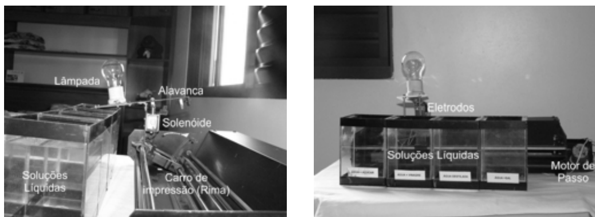
Figura 6 – Estrutura mecânica do experimento Correntes Elétricas em Soluções líquidas
