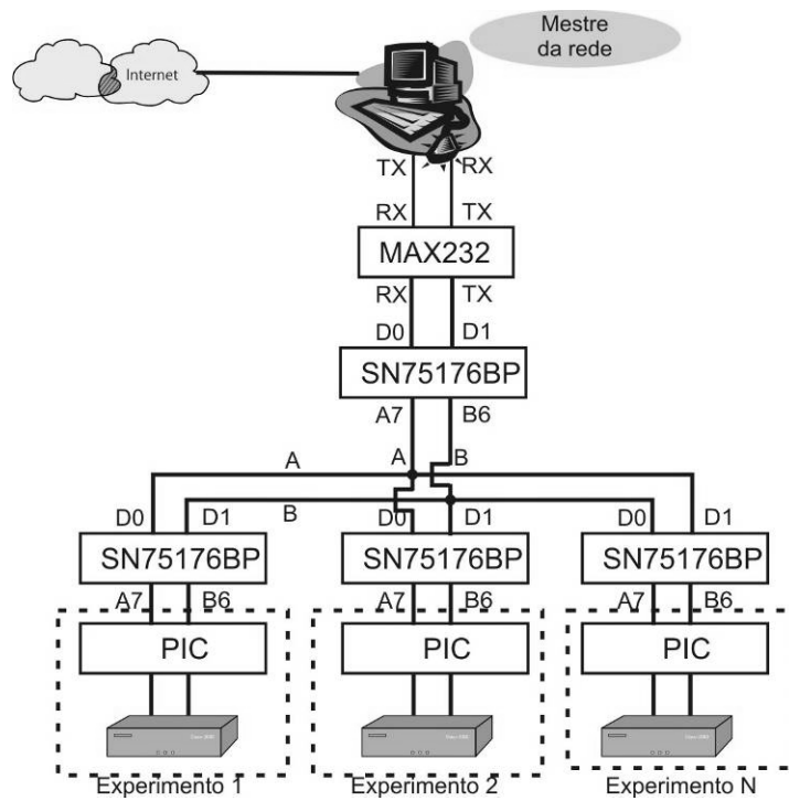
Figura 3 – Rede 485 no projeto WebLab
