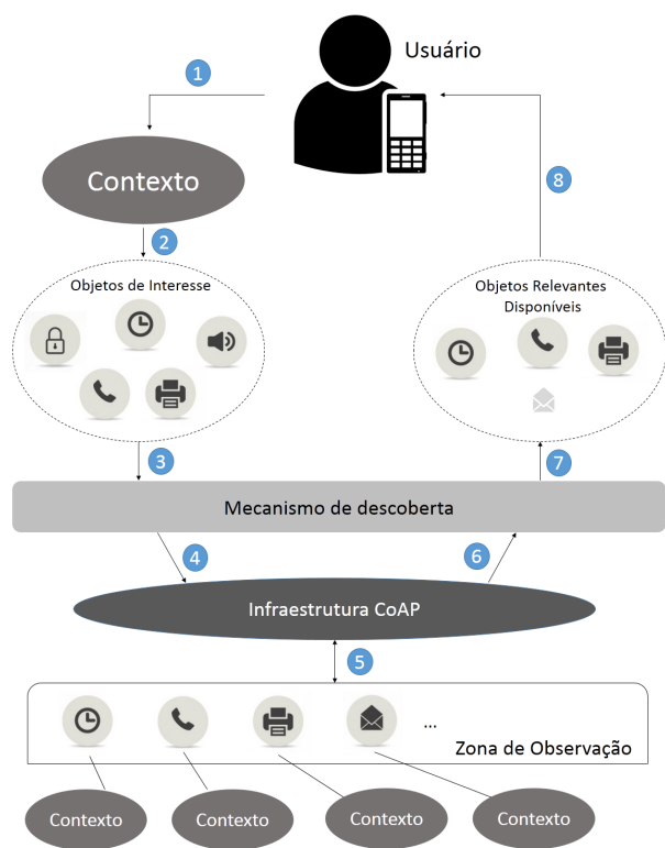
Figura 2: Visão geral do processo de descoberta proposto de objetos inteligentes.
