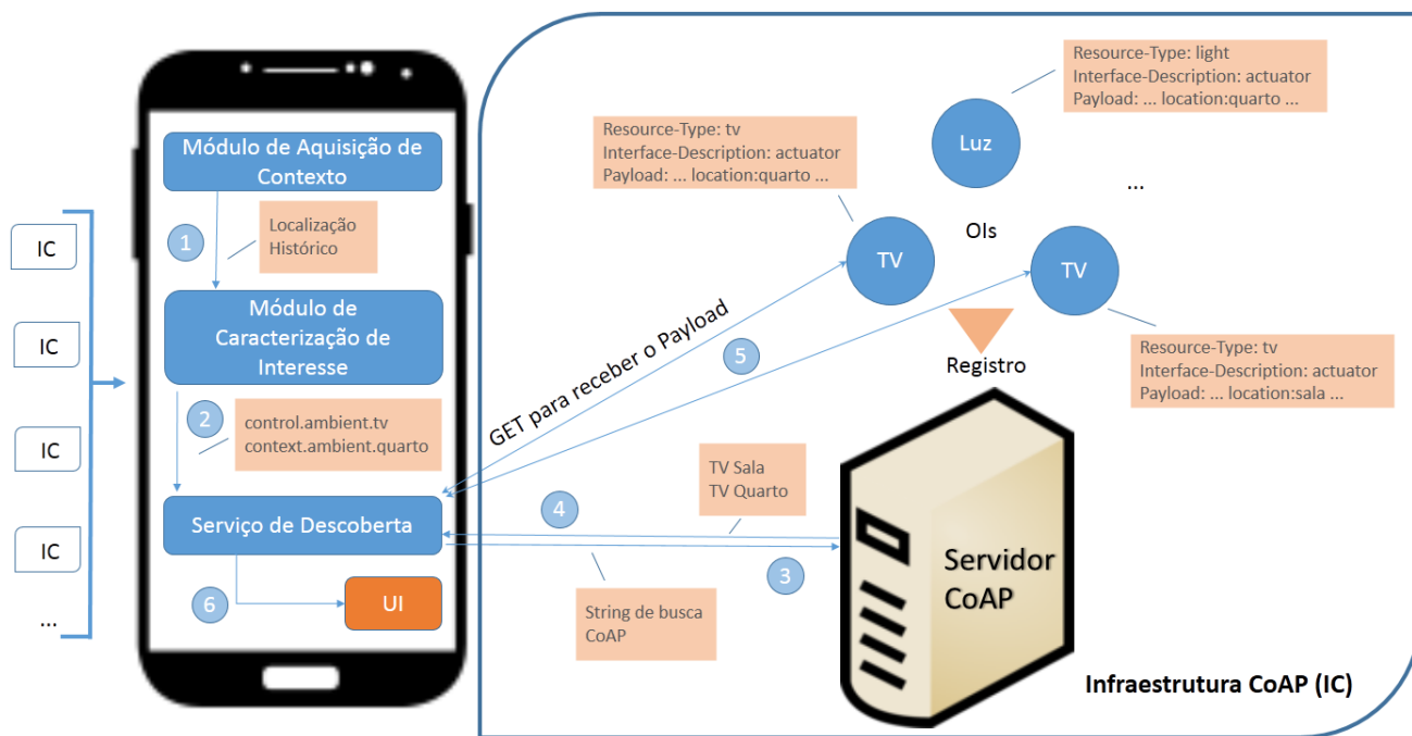
Figura 3: Exemplo de utilização do processo de descoberta proposto em um cenário real de IoT.
