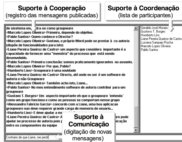
Figura 1. Elementos 3C em um sistema de bate-papo [8]
