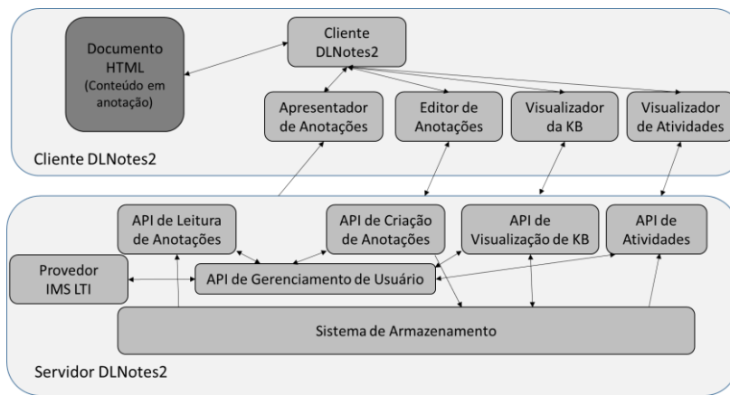
Figura 1. Arquitetura simplificada da DLNotes2
