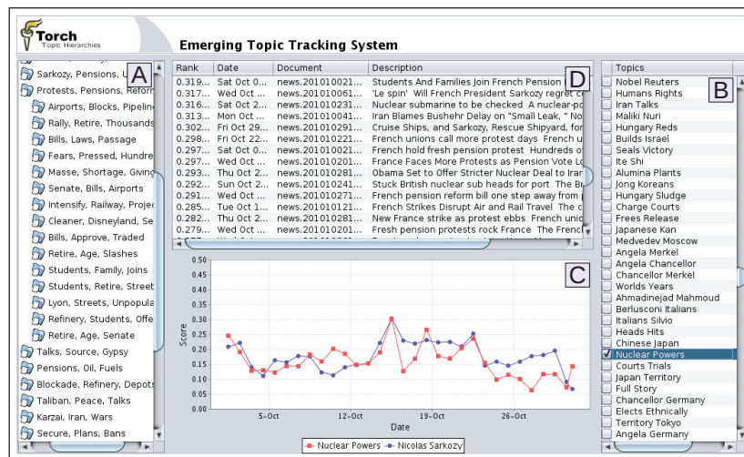
Figura 3: Interface de análise exploratória da Torch-ETS
