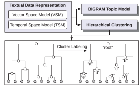
Figura 2: Módulo de mineração temporal dos textos
