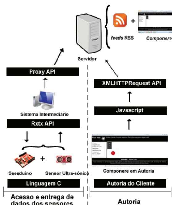
Figura 1: Arquitetura da ferramenta desenvolvida
