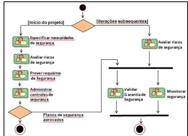
Figura 2. Diagrama de atividade UML com as atividades de segurança
