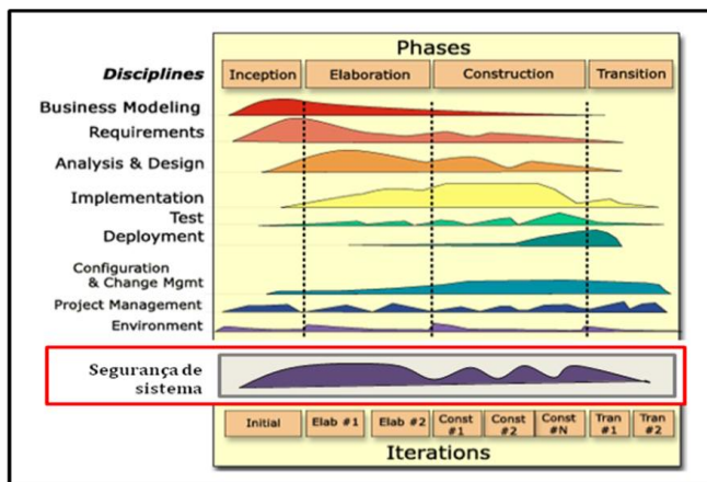
Figura 1. RUP adaptado com a disciplina de segurança
