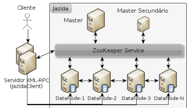
Figure 2: Componentes e arquitetura do Jazida
