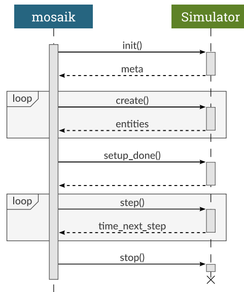
Figura 2. Sequencia de mensagens enviadas entre Mosaik e processo de simulação.
