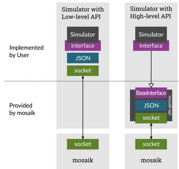
Figura 1. Modelo de API Mosaik de alto nível e de baixo nível.
