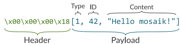
Figura 3. Estrutura das mensagens definidas pelo Mosaik para coordenação e sincronismo no ambiente de co-simulação.
