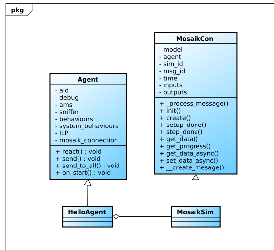
Figura 5. Diagrama de classes UML.
