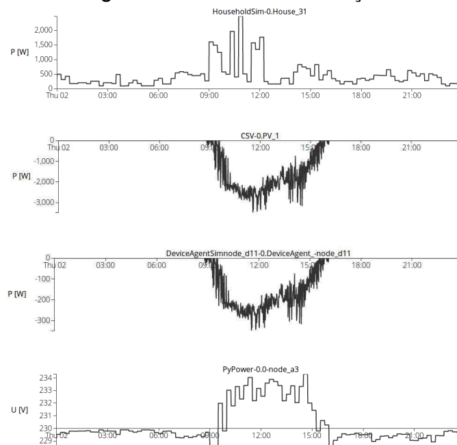
Figura 8. Resultados da simulação.
