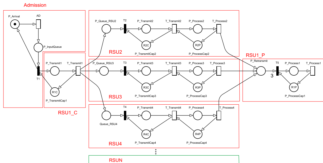
Figura 2. Modelo SPN para o cenário VANET
