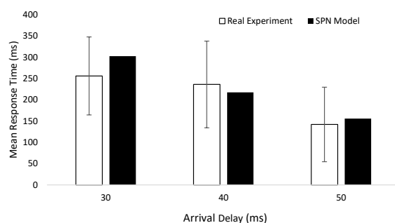
Figura 5. Comparação entre os MRTs do Modelo e do Experimento
