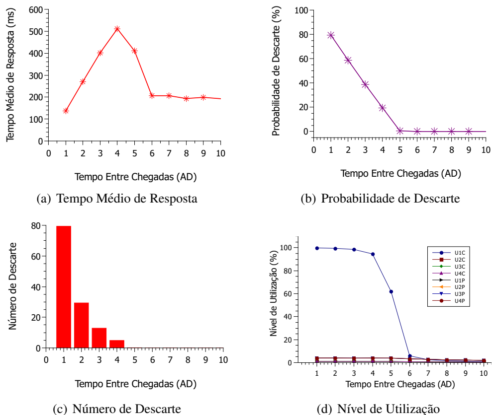
Figura 3. Resultados da Análise Numérica Variando Tempo entre Chegadas
