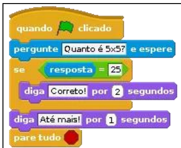
Figura 2. Blocos lógicos do Scratch.
