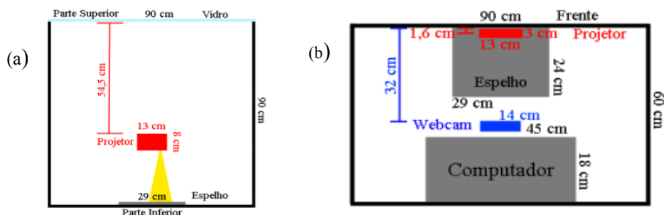
Figura 1. Posicionamento dos componentes físicos do artefato
