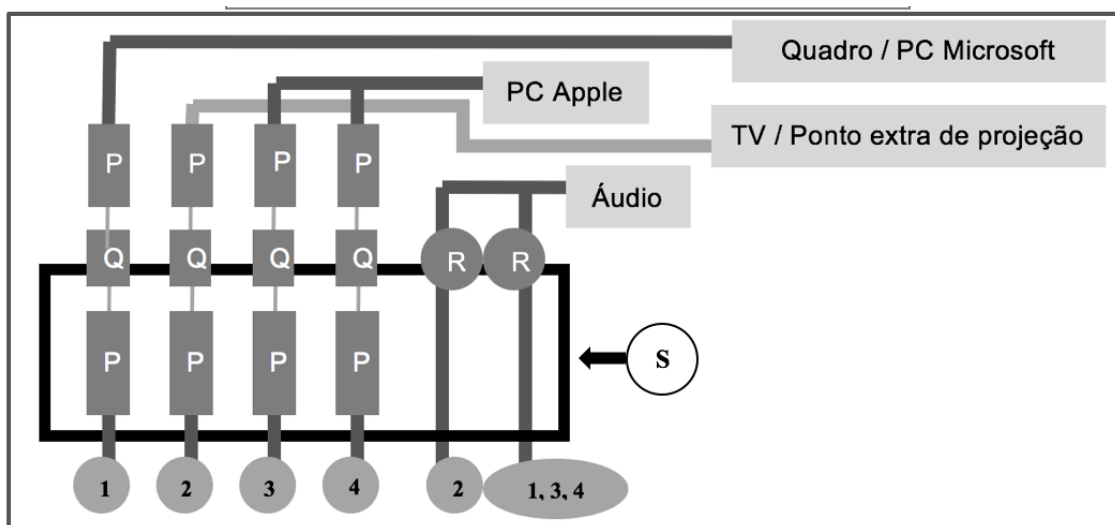
Figura 9 - Dispositivo centralizador de Áudio e Vídeo
