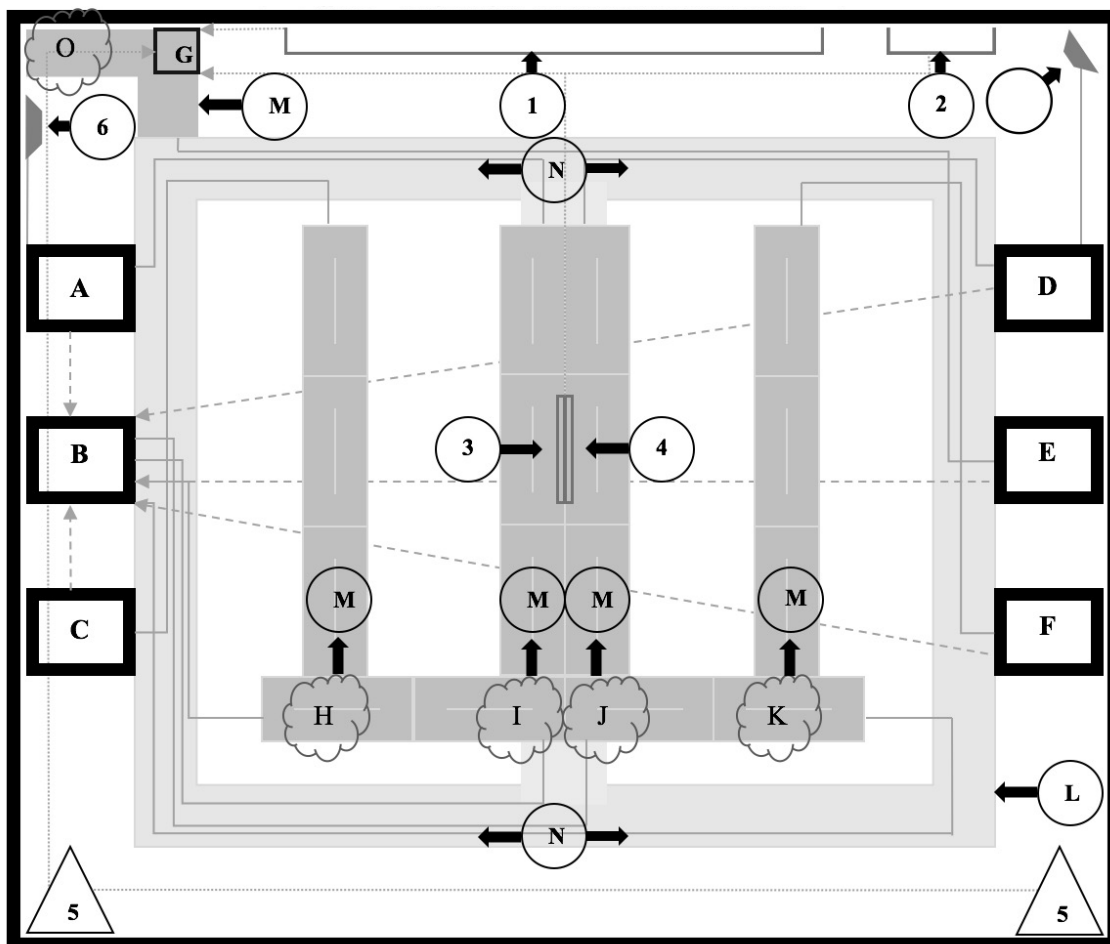
Figura 7 - Planta dos elementos do LADIR
