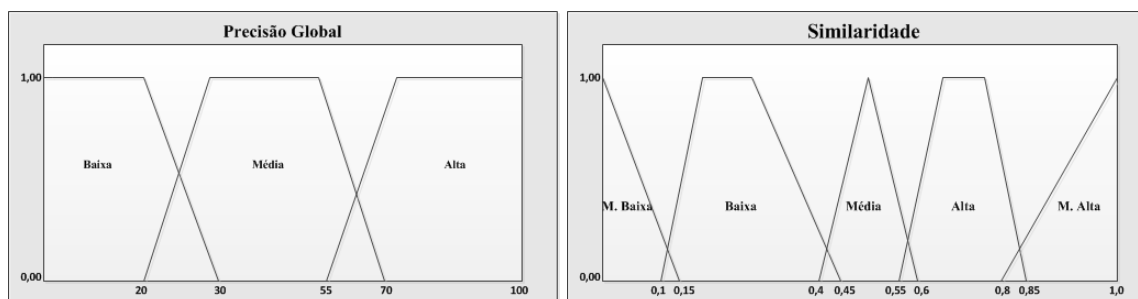
Figura 2. Gráficos das variáveis linguísticas precisão global e similaridade
