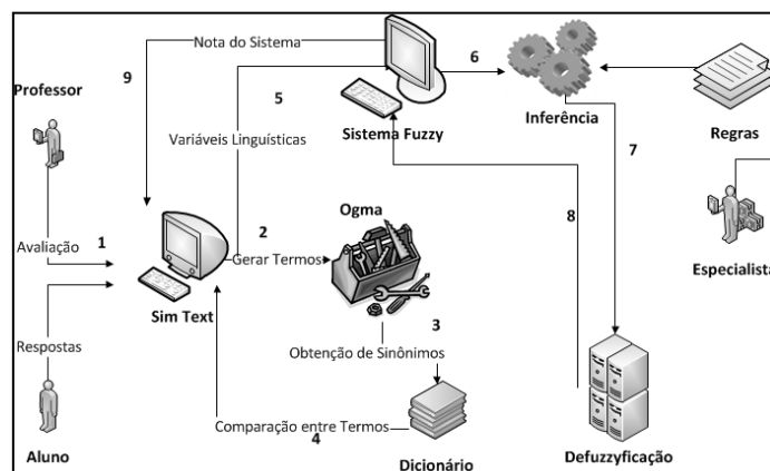
Figura 1. Arquitetura e Funcionamento do Sistema SCATeDi
