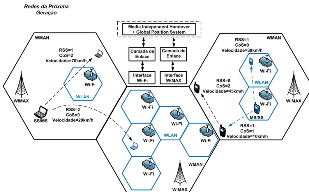
Figura 2. Arquitetura do MIH2Q em Redes Heterogêneas da Próxima Geração
